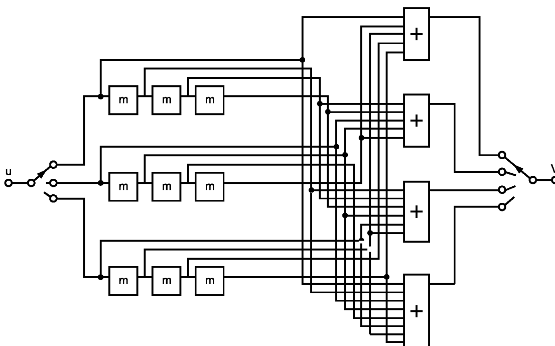
Рисунок К.1 — Схема кодирования со структурой 4-3-3 для символа уровня ECC 050
