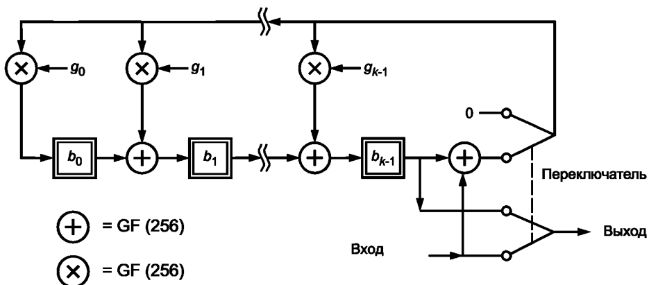
Рисунок 5 — Схема генерации кодовых слов исправления ошибки
