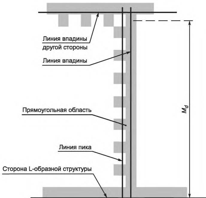
Рисунок 11 — Построение прямоугольной области
