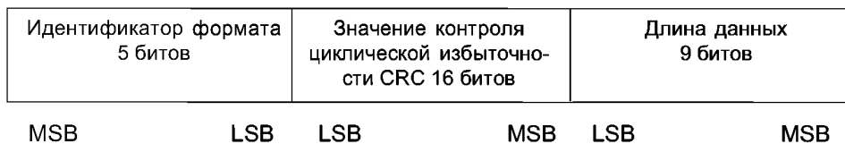
Рисунок 8 — Структура префикса двоичного потока данных
