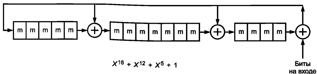
Рисунок J.1 — Схема алгоритма расчета CRC
