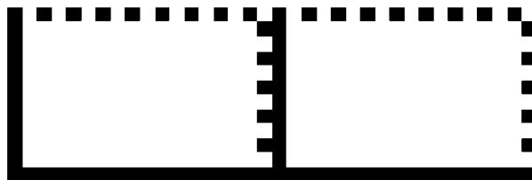
Рисунок D.4 — Конфигурация направляющего шаблона для символа прямоугольной формы 12 × 36 модулей
